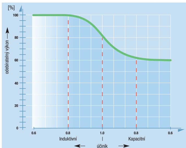
Obr. 8: Závislost odejíratelného výstupního výkonu na velikosti účinníku zátěže
